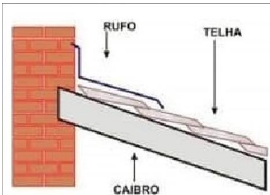
Figura3-Detalhamento do rufo
